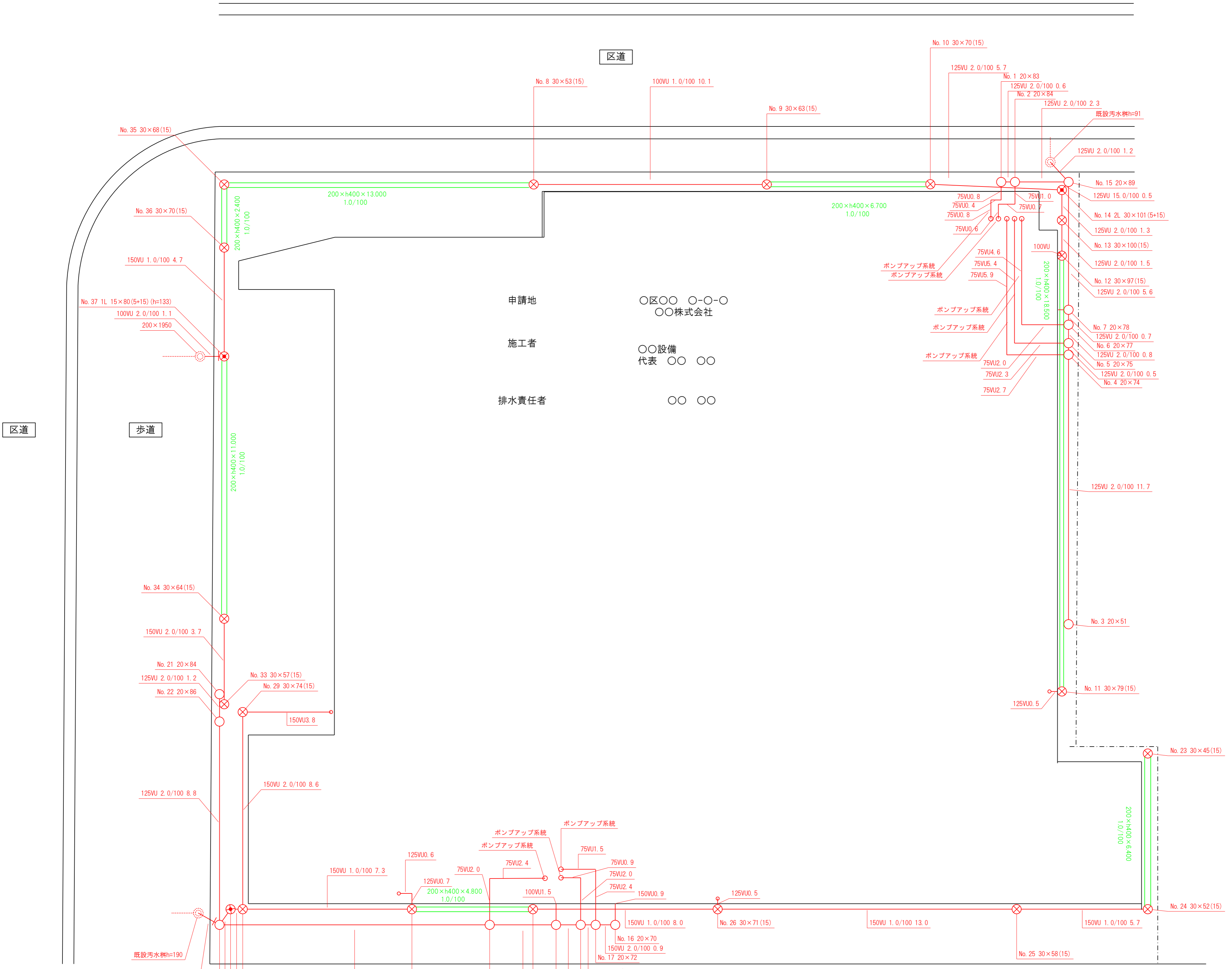
1階 平面図
